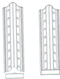
РИС. 1. Установка подпятника на стойку
